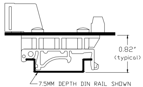
DIN Clip Mounting Option
