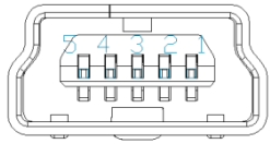
Figure 12: Mini USB Connector
